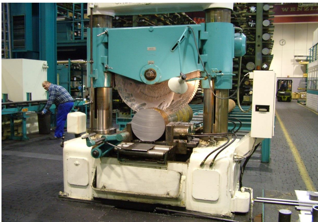
Slika. 4. Kružno piljenje [6]
