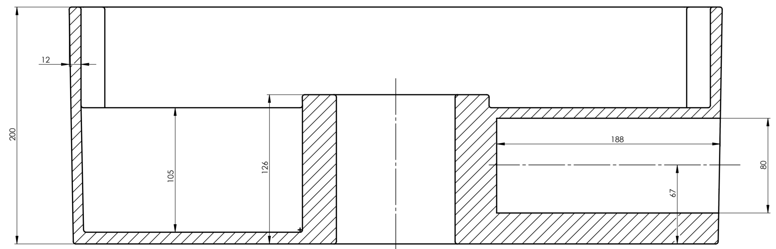
PRESJEK A-A (M 1:1)
