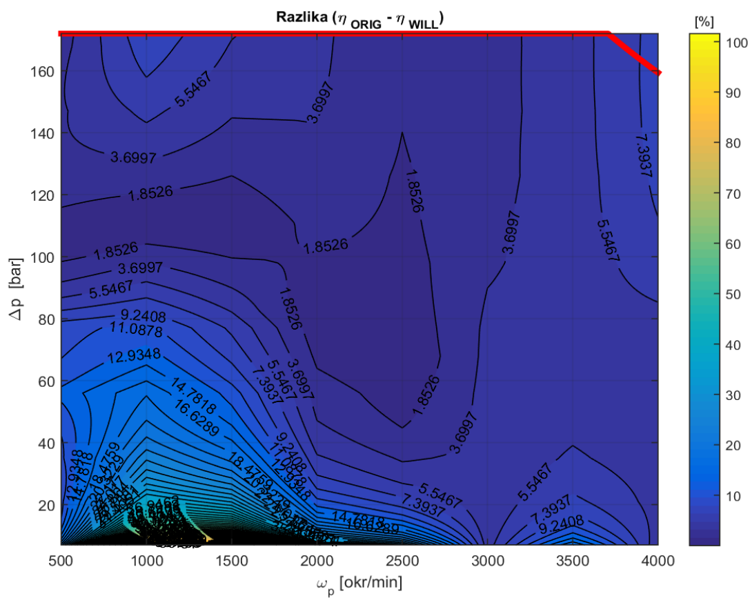
Slika 8.16 Razlika originalne i aproximirane karakteristike, s_p = 0.51
