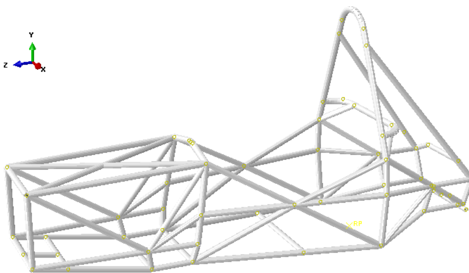
Slika 9. Proračunski model
