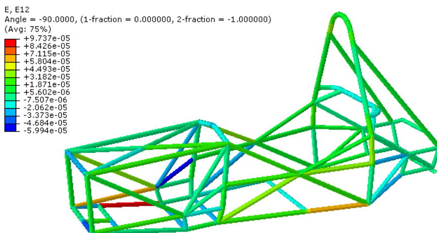
Slika 17. Raspodjela posmičnih deformacija
