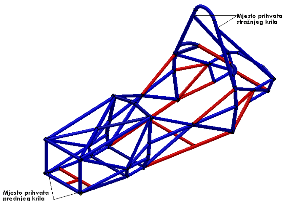
Slika 10. Mjesta prihvata krila i ovješene masa
