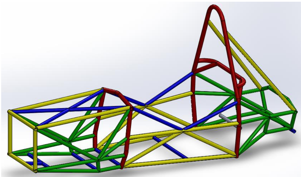
Slika 1. Podvozje
