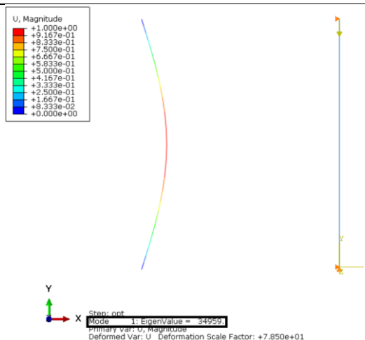
Slika 41. Prikaz rezultata izvijana za drugi primjer
