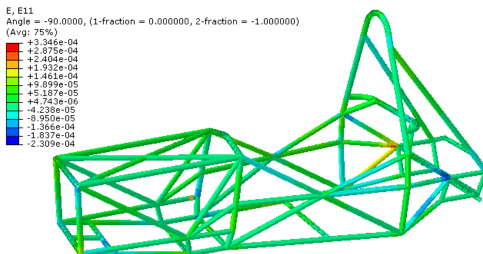
Slika 35. Duljinske deformacije
