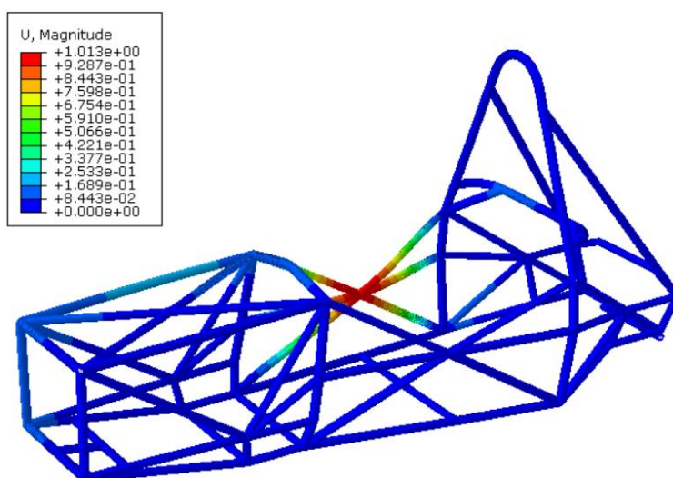
Slika 45. Gubitak stabilnosti pri skretanju (prva vlastita vrijednost)
