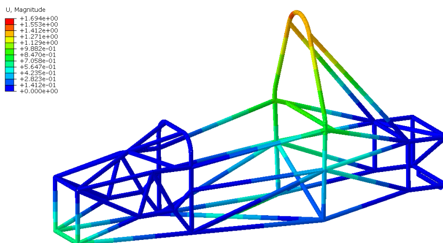
Slika 52. Raspodjela rezultantnog pomaka na prethodnom podvozju pri kočenju
