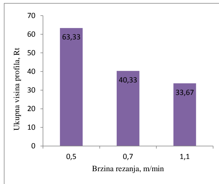
Slika 38. Prikaz ovisnosti ukupne visine profila (Rt) i brzine rezanja (debljina 10 mm)
