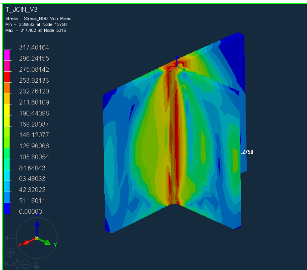
Slika 30. Raspored napreznja, T_p= 250^{\circ}\text{C}
