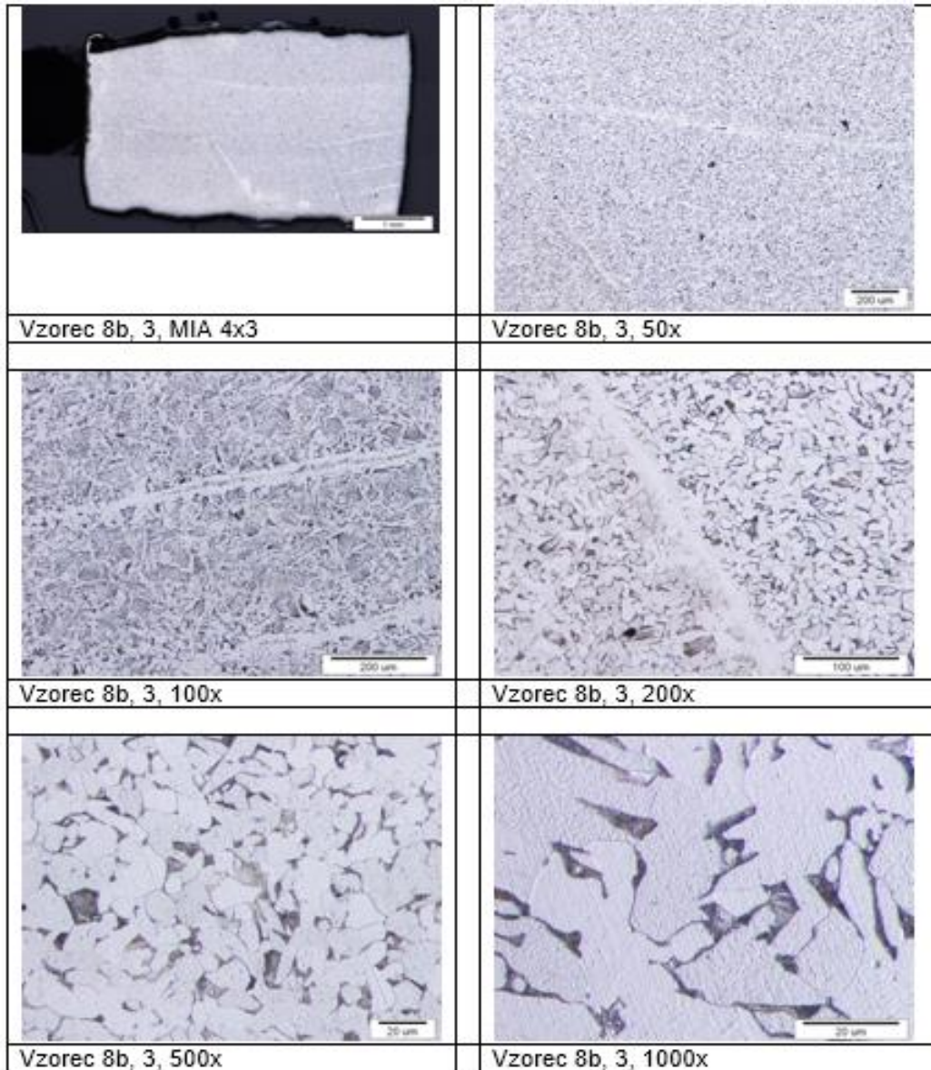
Slika 5.5: Mikrostruktura dijela 8b.3
