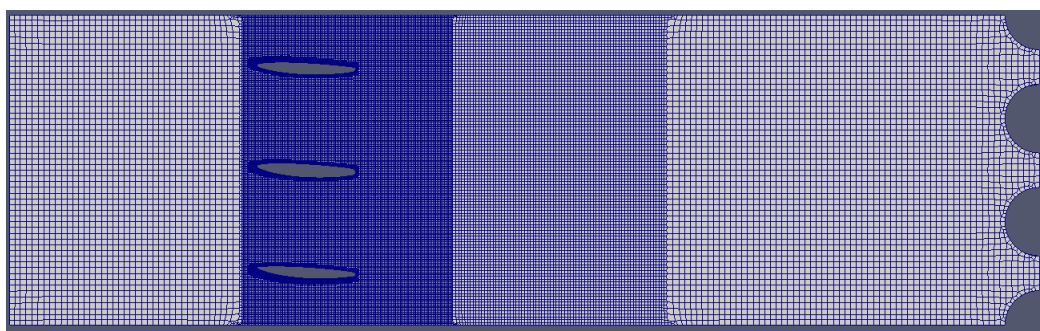
Slika 4.8: Prikaz mreže s tri lopatice
