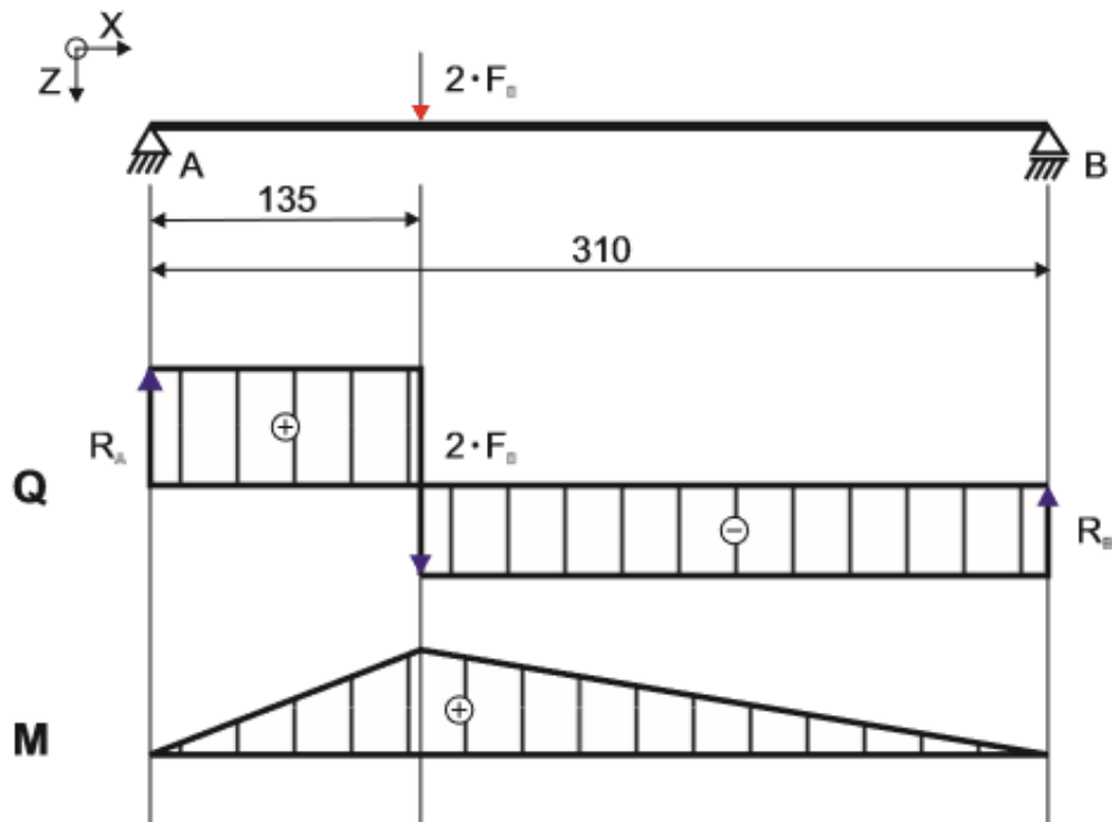
Slika 10: Opterećenje i dijagrami unutarnjih sila međuvratila
