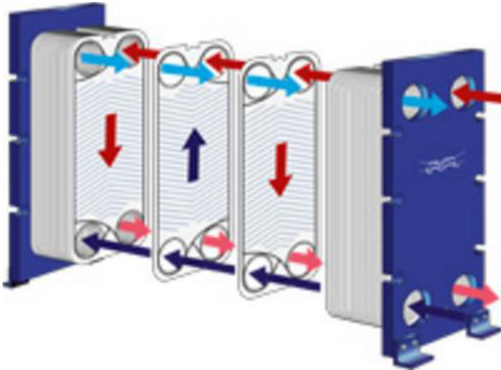
Slika 9. Kompaktni pločasti isparivač
