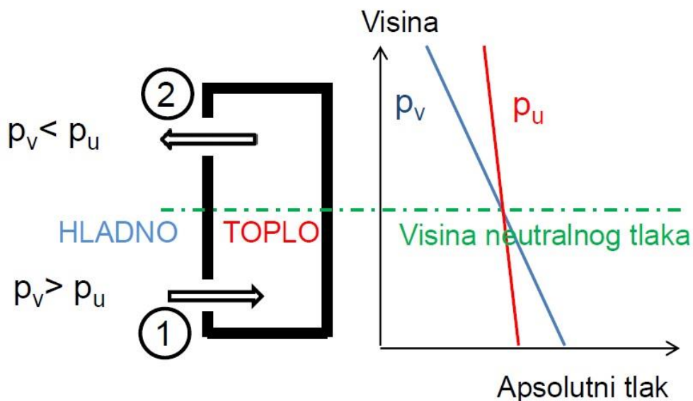
Slika 2. Razdioba tlaka vanjskog okoliša i unutarnjeg prostora [1]
