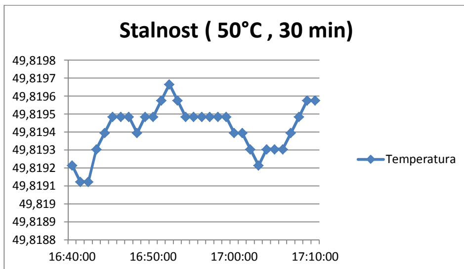
Slika 18: Stalnost temperature za 50°C - kupka Kambič/voda
