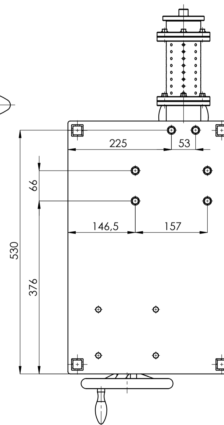
A-A (1:5)
