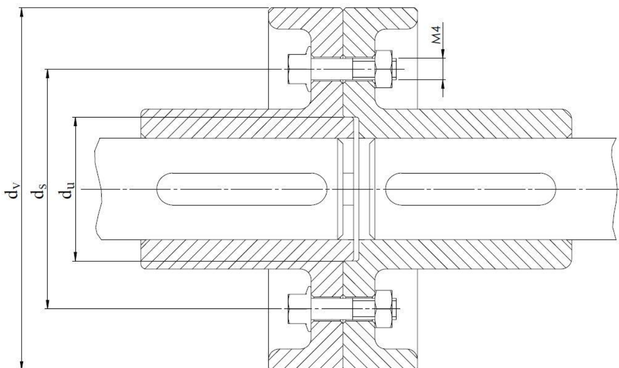
Slika 28. Kolutna spojka
