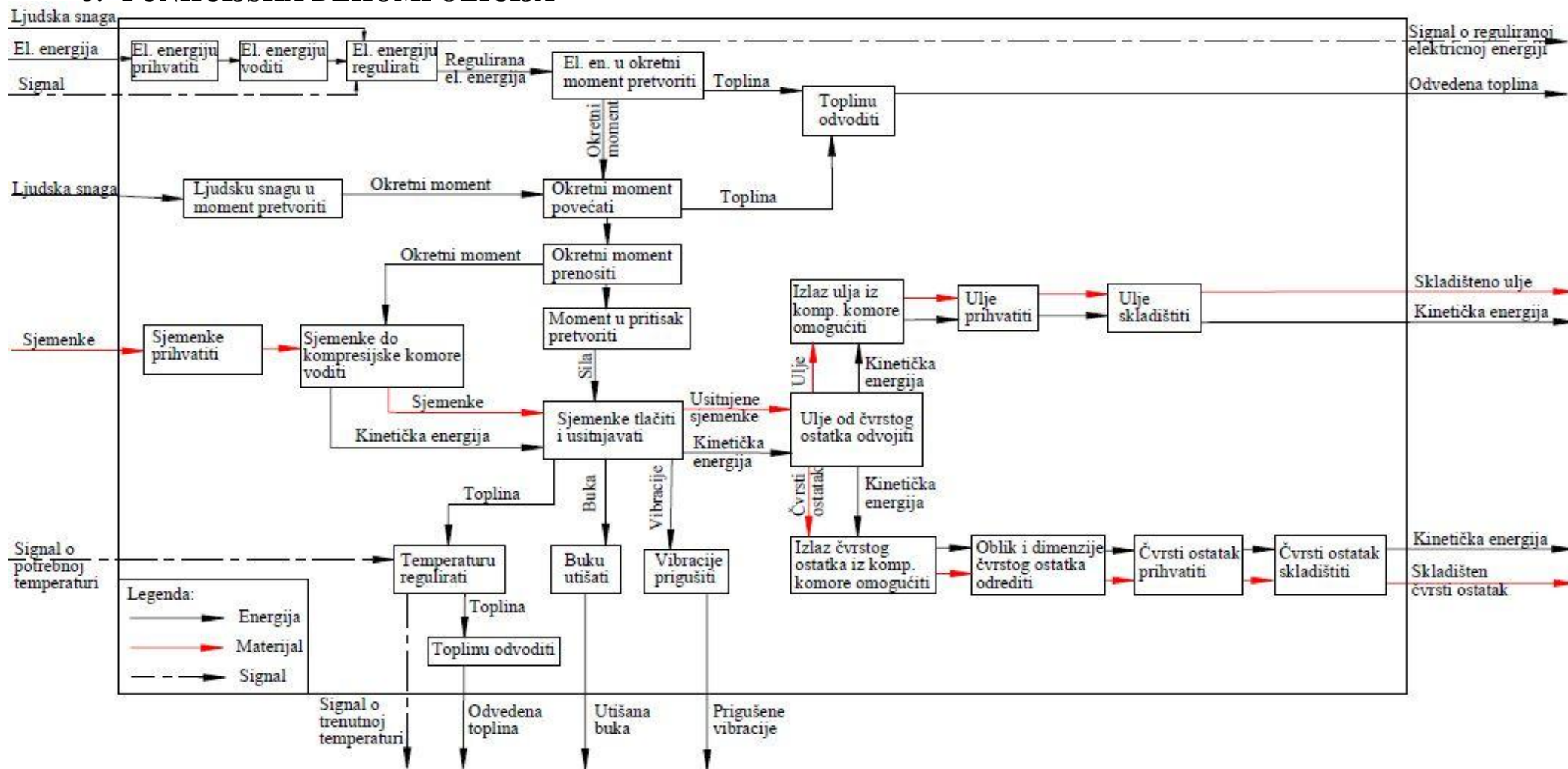
Slika 11. Funkcijska dekompozicija
