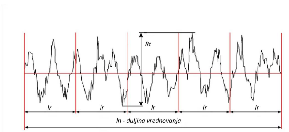
Slika 19. Ukupna visina profila R_t
