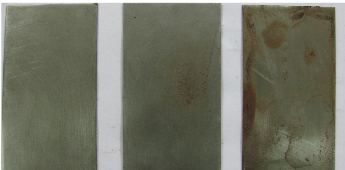
Slika 24. Rezultati ispitivanja uzoraka od čelika PE folijom debljine 100 \mu\text{m} u slanoj komori
