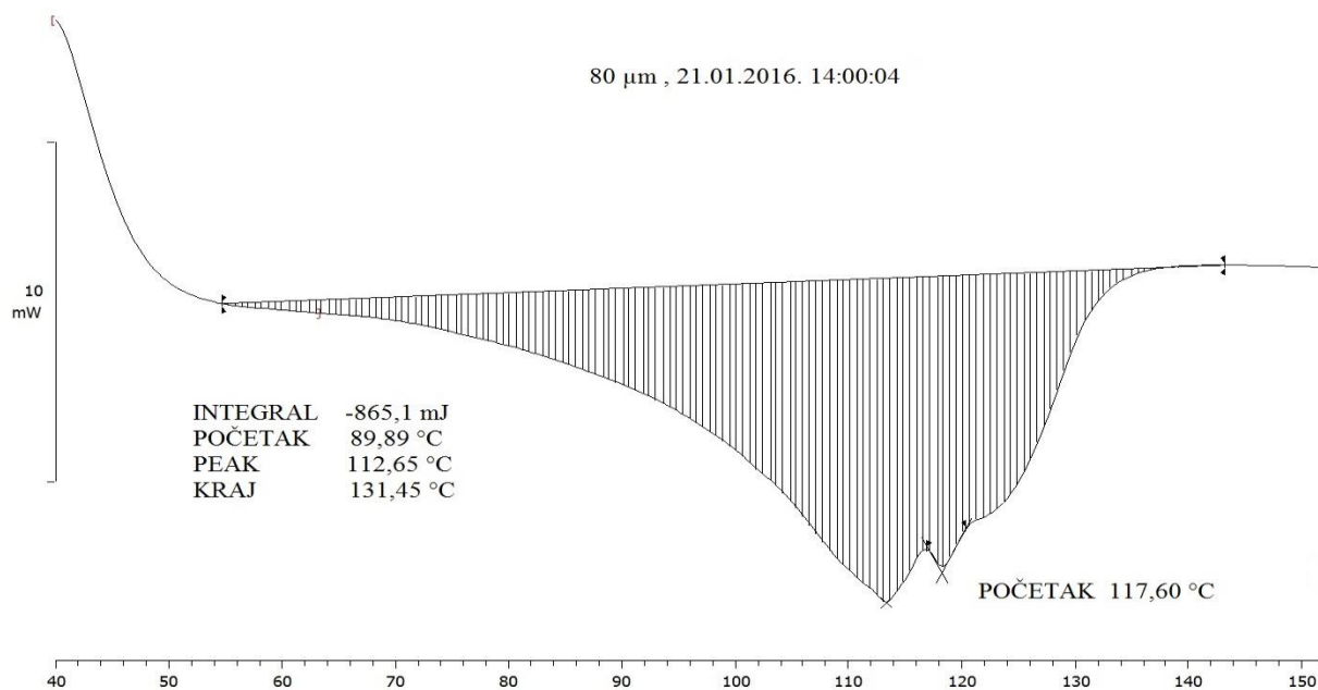
Slika 43. DSC krivulja za uzorak PE folije od 80 μm
