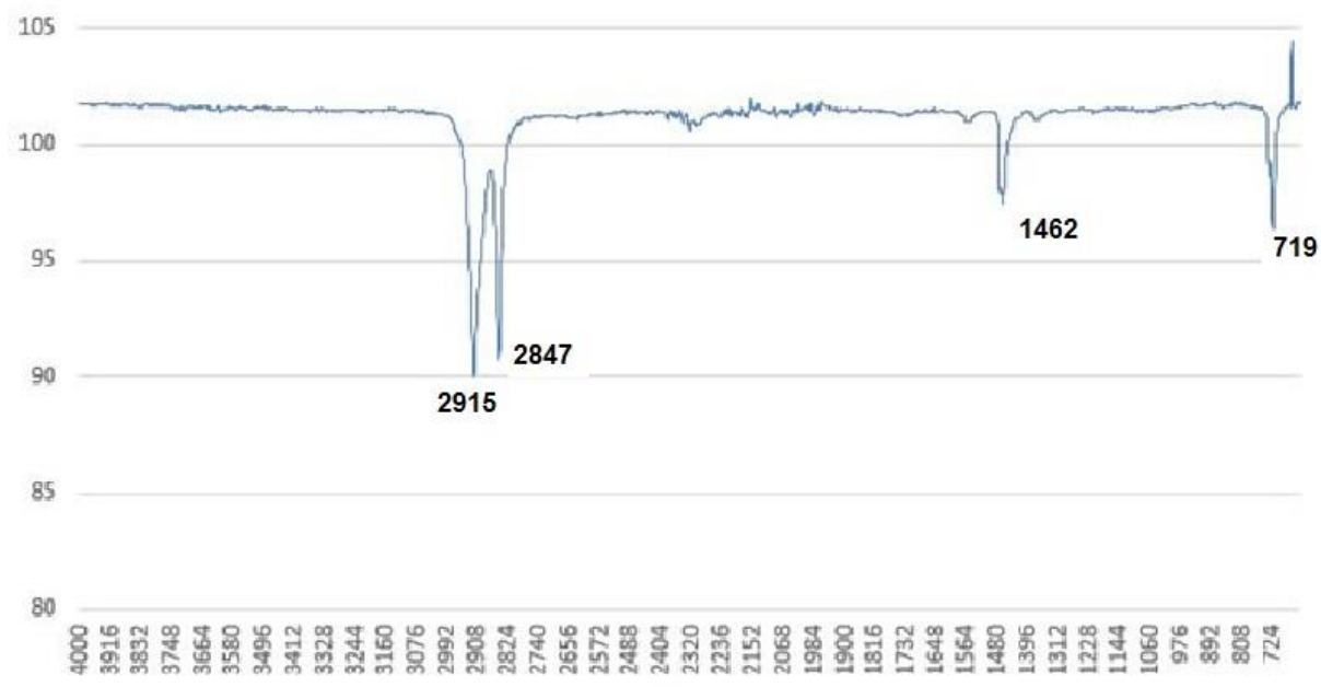
Slika 47. FTIR spektr PE folije od 80 \mu\text{m} , 100 \mu\text{m} i 120 \mu\text{m} s vanjske strane
