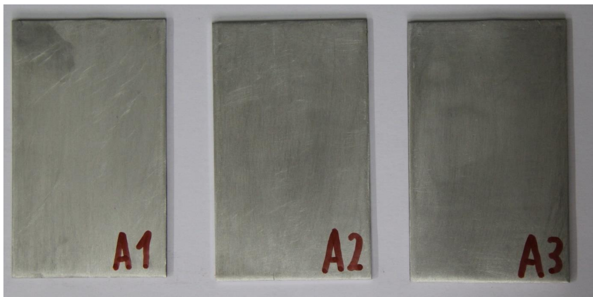
Slika 36. Rezultati ispitivanja uzoraka od čelika PE folijom debljine 120 \mu\text{m} u vlažnoj komori
