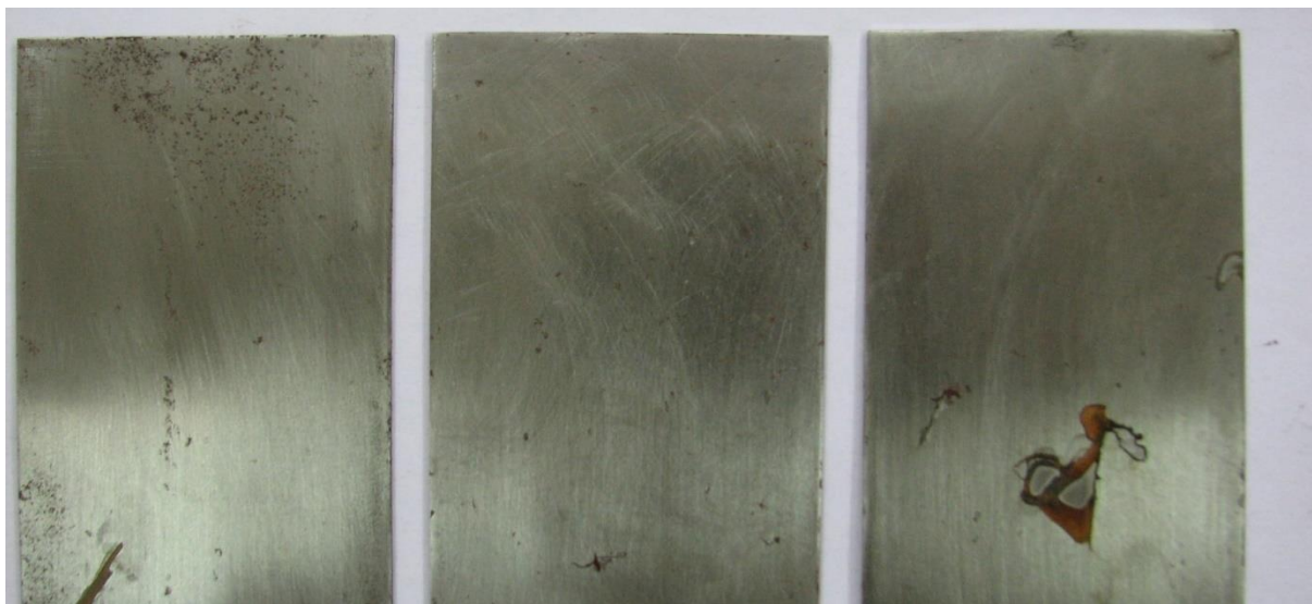
Slika 19. Rezultati ispitivanja uzoraka od čelika PE folijom debljine 80 \mu\text{m} u slanoj komori
