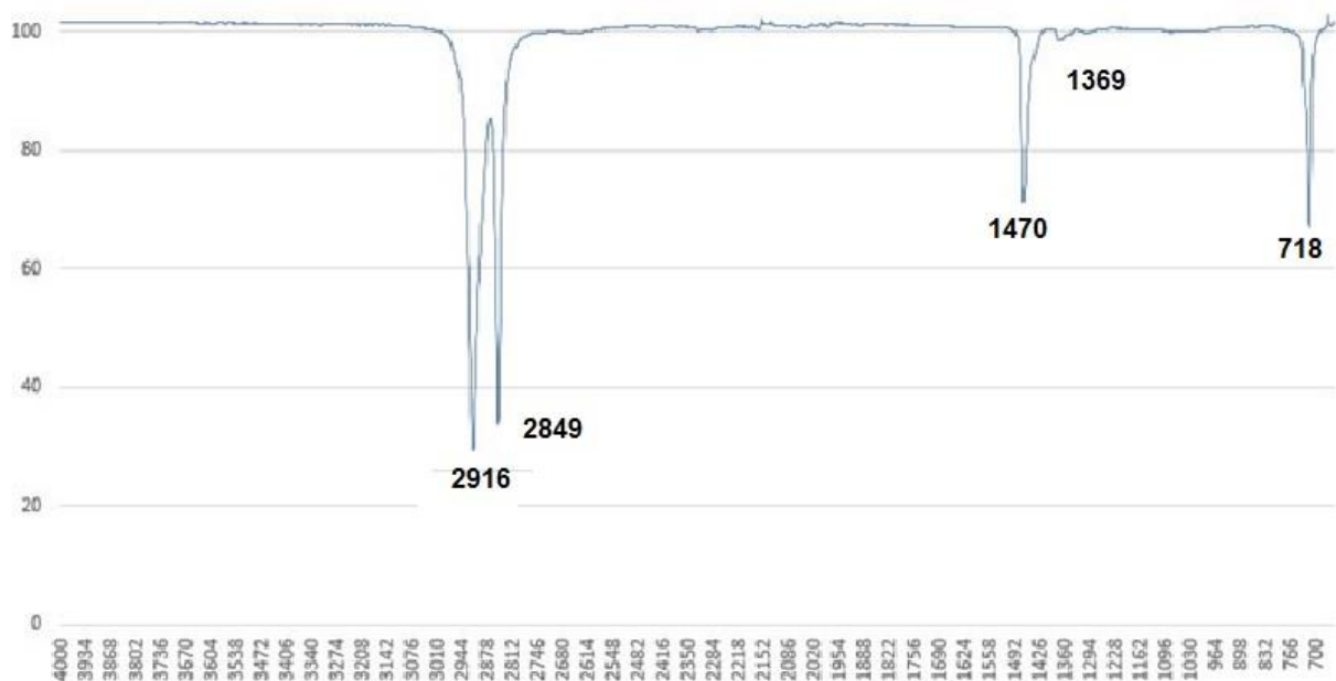
Slika 48. FTIR spektr PE folije od 80 \mu\text{m} sa stane inhibitora
