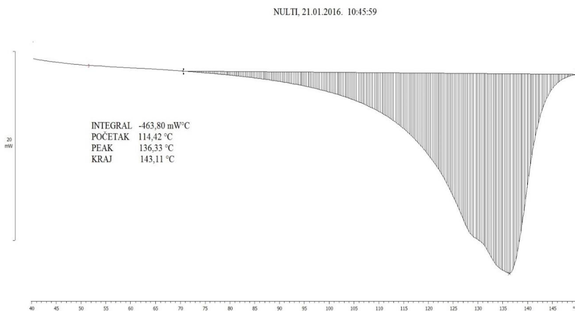
Slika 42. DSC krivulja za uzorak nulte probe
