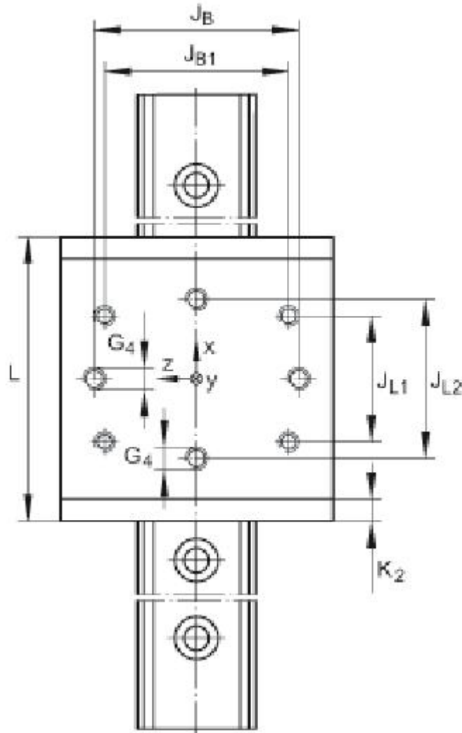
Slika 29 Uzdužna vodilica
