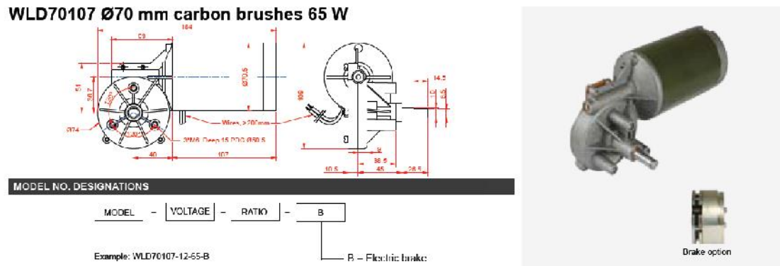
Slika 27 Odabrani elektromotor za pogon uzdužnih kliza a
