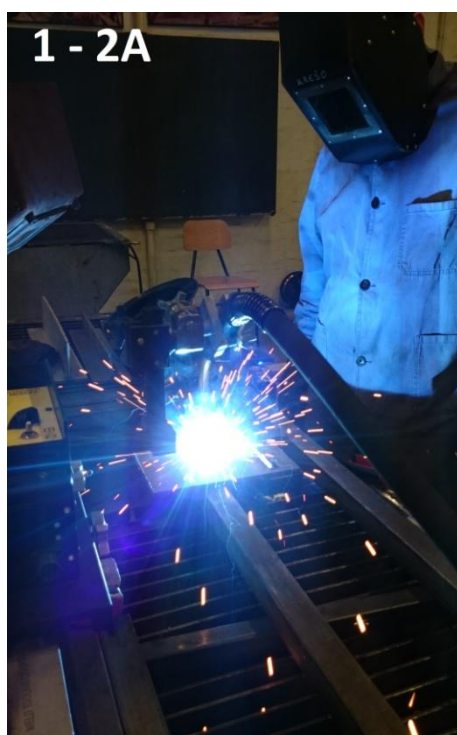
Slika 31. Navarivanje strujom 175 A i plinskom mješavinom Ferroline C6 X1
