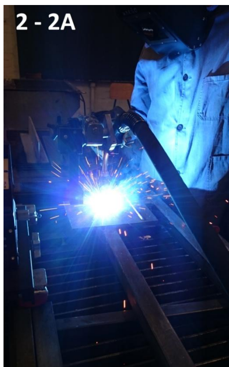
Slika 31. Navarivanje strujom 175 A i plinskom mješavinom Ferroline C6 X1
