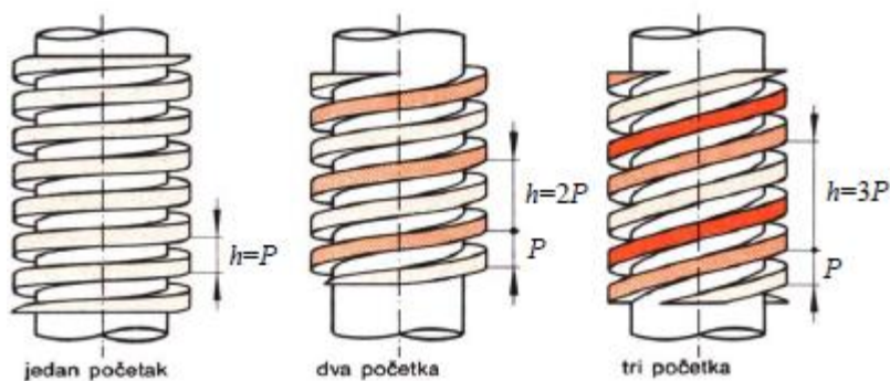
Slika 2. a) jednovojni navoj, b) dvovojni navoj, c) trovojni navoj
