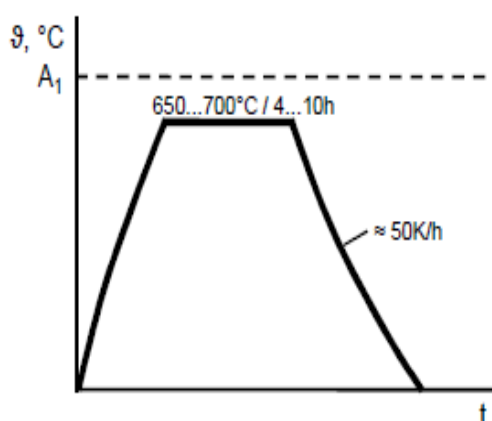
Slika 2.3. Žarenje za redukciju zaostalih napreznja čelika s 12% Cr [1]
