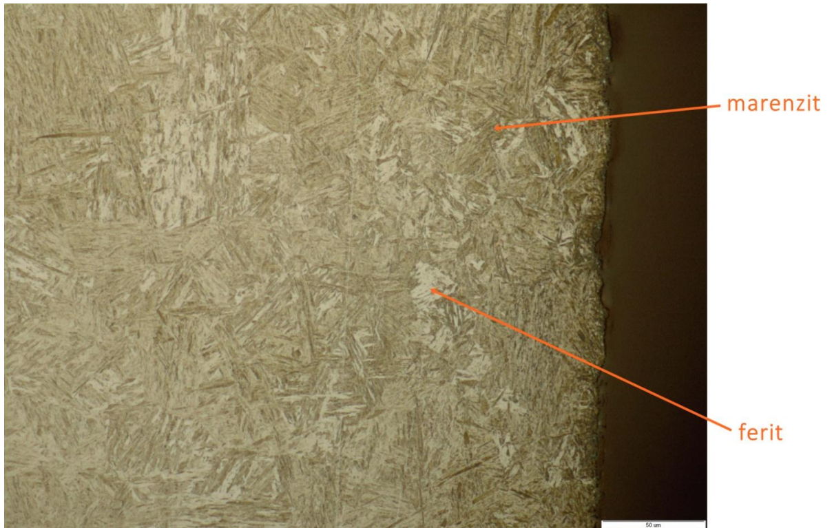
Slika 34. Mikrostruktura uzorka 2 u nagriženom stanju, povećanje 500x
