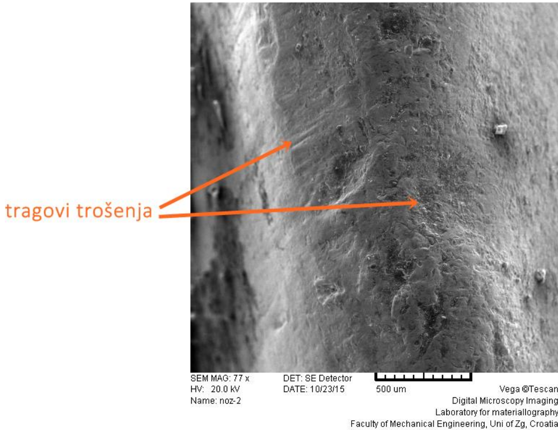
Slika 27. Prikaz oštrice noža snimljene na SEM-u
