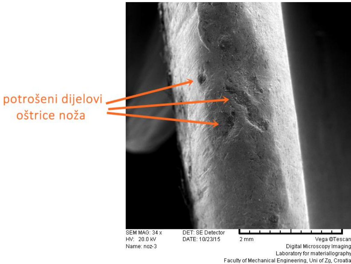
Slika 28. Prikaz oštrice noža snimljene na SEM-u
