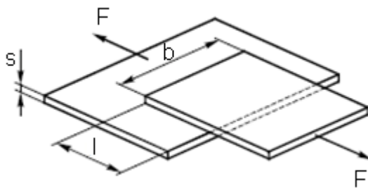
Slika 23. Odnos duljine lijepljenog spoja i debljine osnovnog materijala [4]
