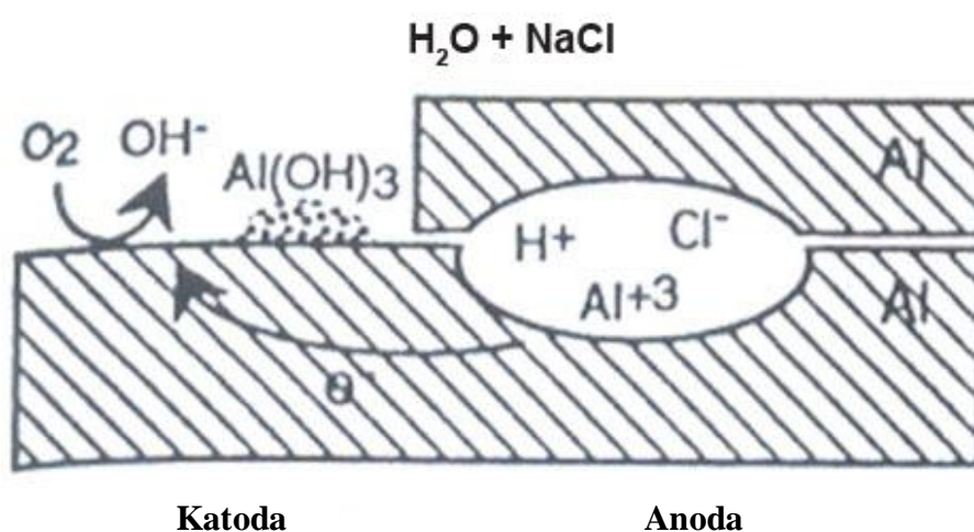
Slika 6. Korozijska u procijepu aluminijska [8]
