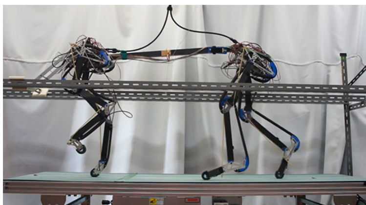
Slika 9: Trčeći pneumatski robot-PNEUPARD [7]
