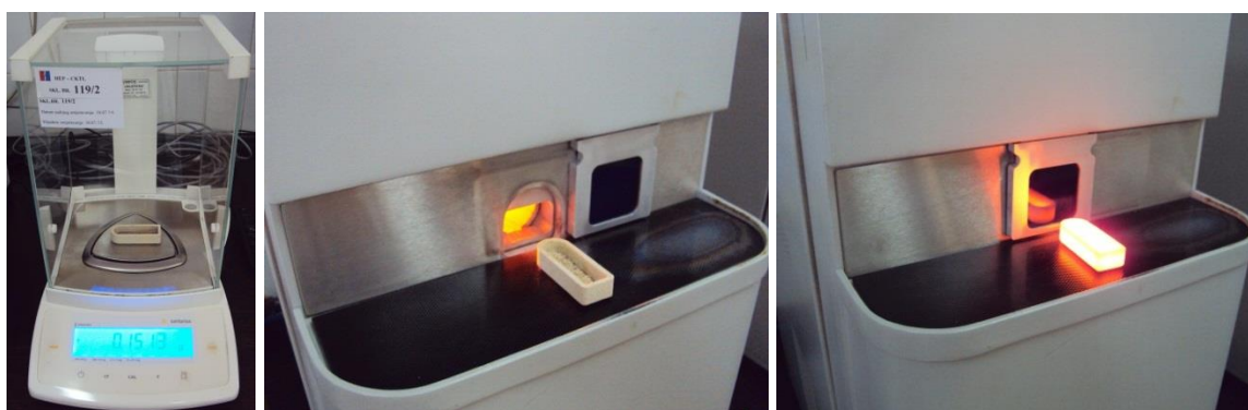
Slika 55. Vaganje lađice s uzorkom (lijevo), lađica s uzorkom prije (lijevo) i nakon (desno) analize sumpora
