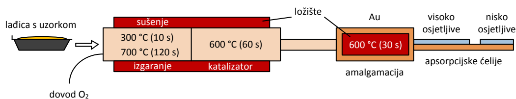
Slika 40. Pojednostavljeni prikaz rada automatskog analizatora žive [20]
