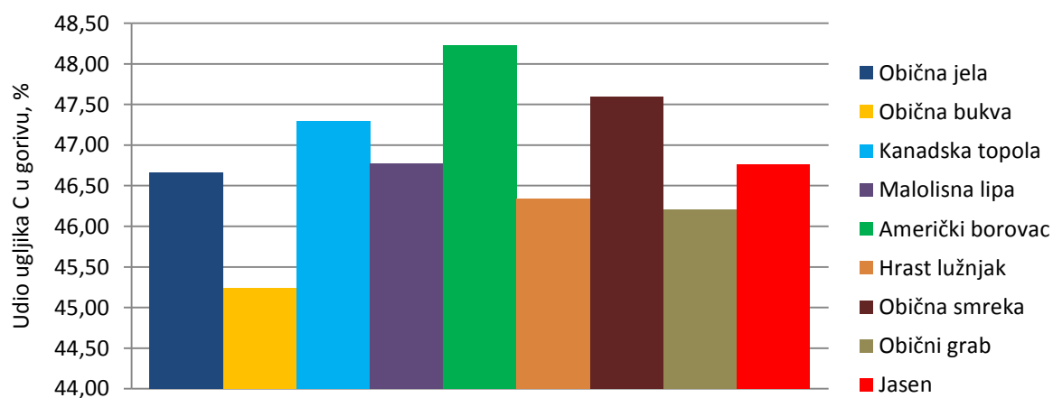
Slika 56. Sadržaj ugljika u pojedinom drvu
