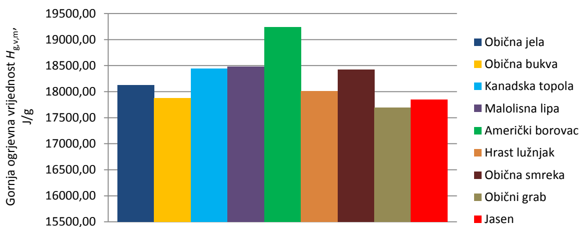
Slika 35. Gornje ogrjevne vrijednosti uzoraka drvene sječke
