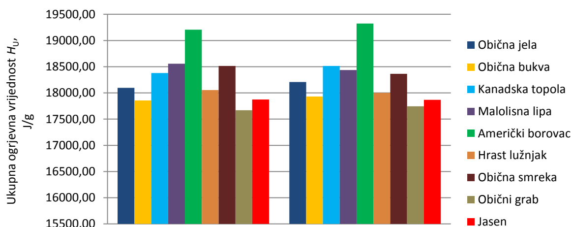
Slika 34. Ukupne ogrjevne vrijednosti uzoraka drvene sječke
