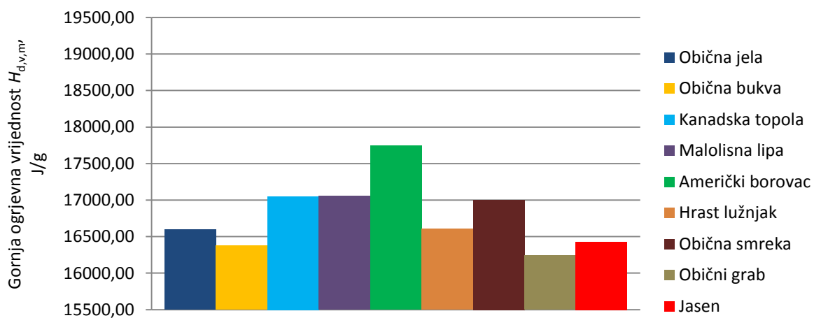
Slika 36. Donje ogrjevne vrijednosti uzoraka drvene sječke
