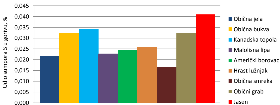
Slika 59. Sadržaj sumpora u pojedinom drvu
