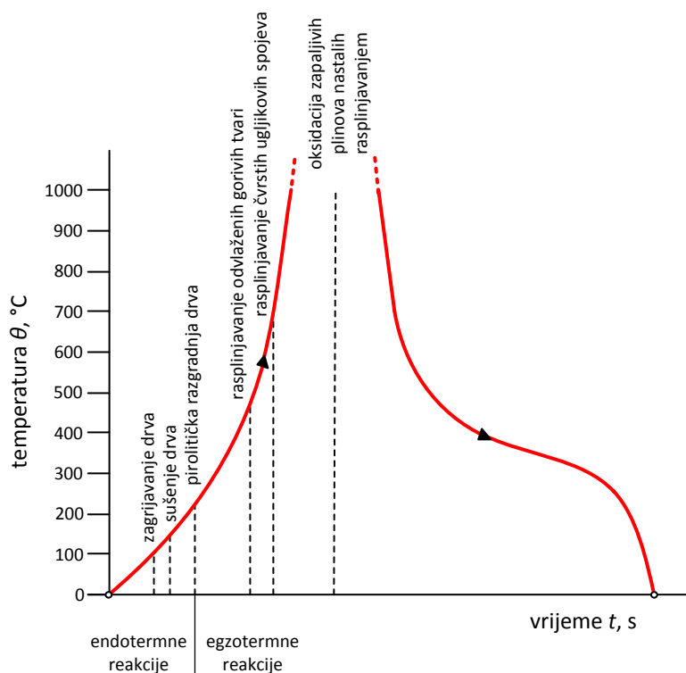
Slika 51. Faze izgaranja biomase [3]
