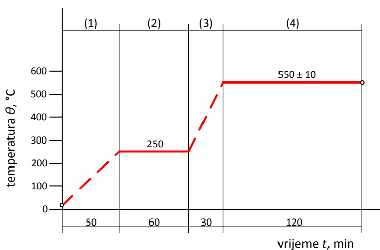
Slika 14. Temperaturni profil žarenja
