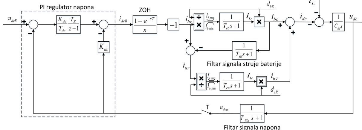
Sl. 42. Regulacijski krug napona DC sabirnice
