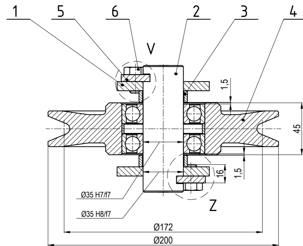
Presjek B-B
