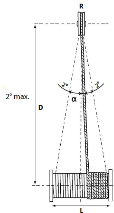
Slika 32: Nagib užeta naspram duljini bubnja [4]
