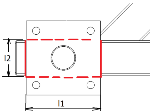
Slika 6.16. Pogled zavara 2
