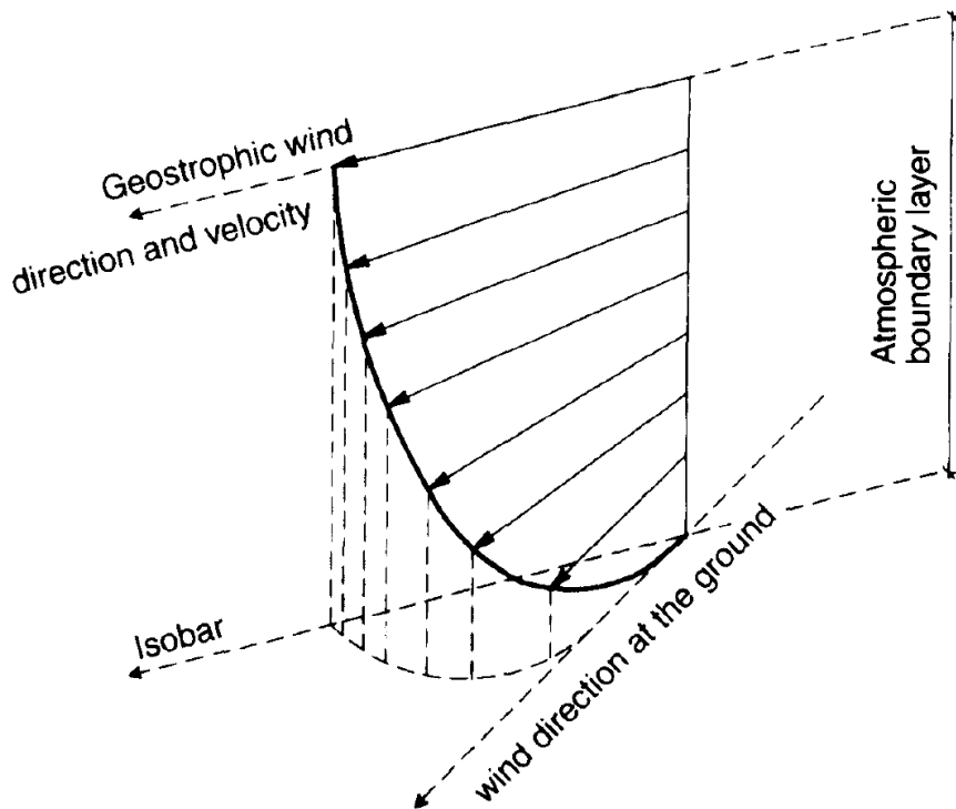
Slika 4: Strujanje zraka u atmosferskom graničnom sloju [6]
