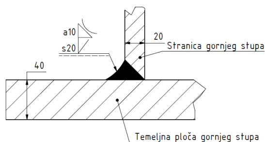
Slika 6.15. Veličina i oblik zavora I
