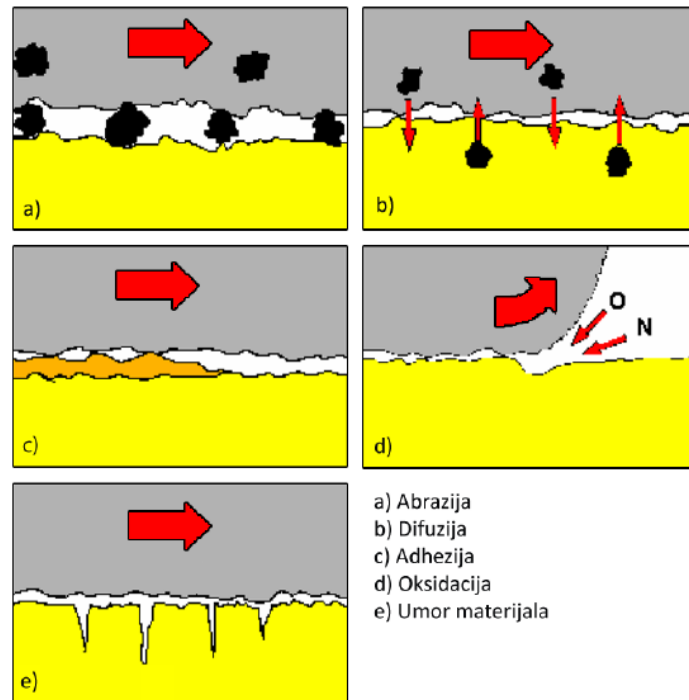
Slika 5.3. Mehanizmi trošenja [28]
