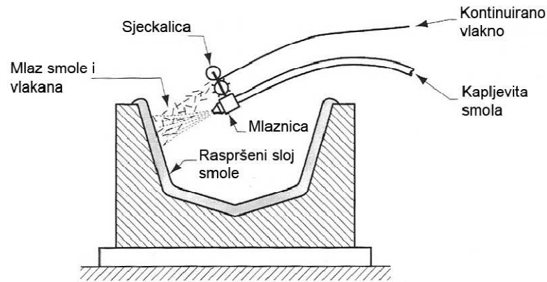
Slika 2.22. Shematski prikaz naštrcavanja [3]
