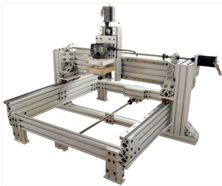
Slika 33. Primjer postolja CNC stroja izrađenog od aluminijskih profila [19]
