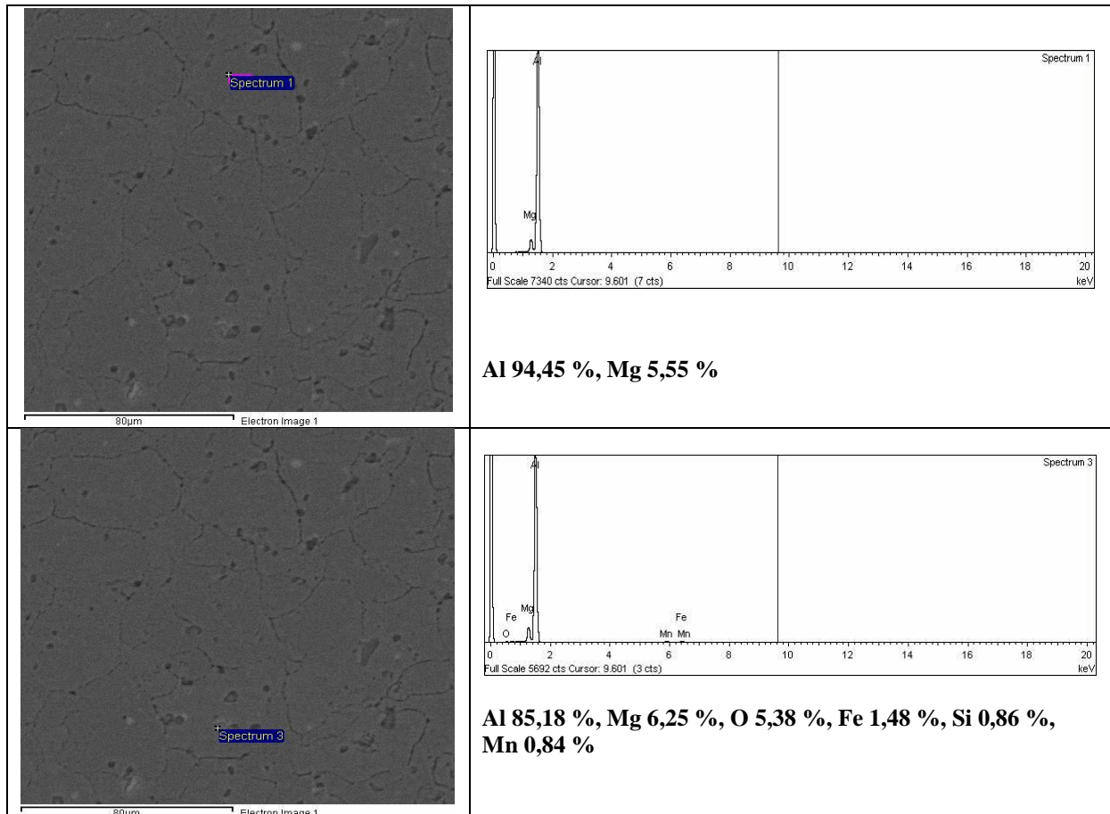
Slika 37. SEM uzorka 1
