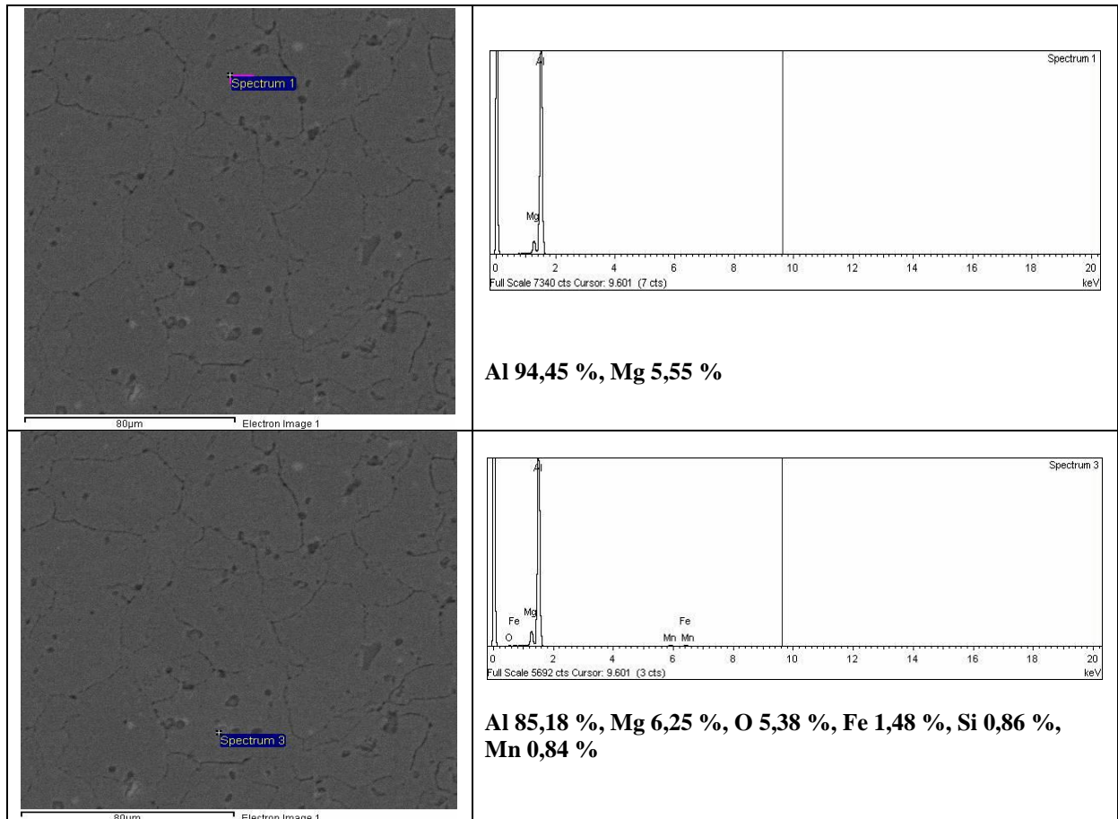
Slika 37. SEM uzorka 1
