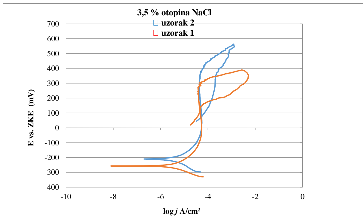
Slika 52. Dijagrami cikličke polarizacije uzorka 1 i 2 u 3,5 % otopini NaCl pri (20\pm 2) °C
