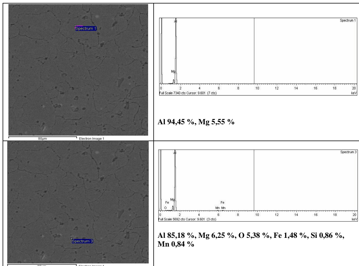
Slika 37. SEM uzorka 1
