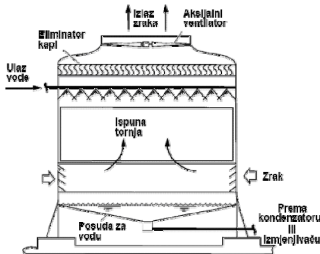
Slika 7.5 Protusmjerni rashladni tornanj s induciranim strujanjem [4]
