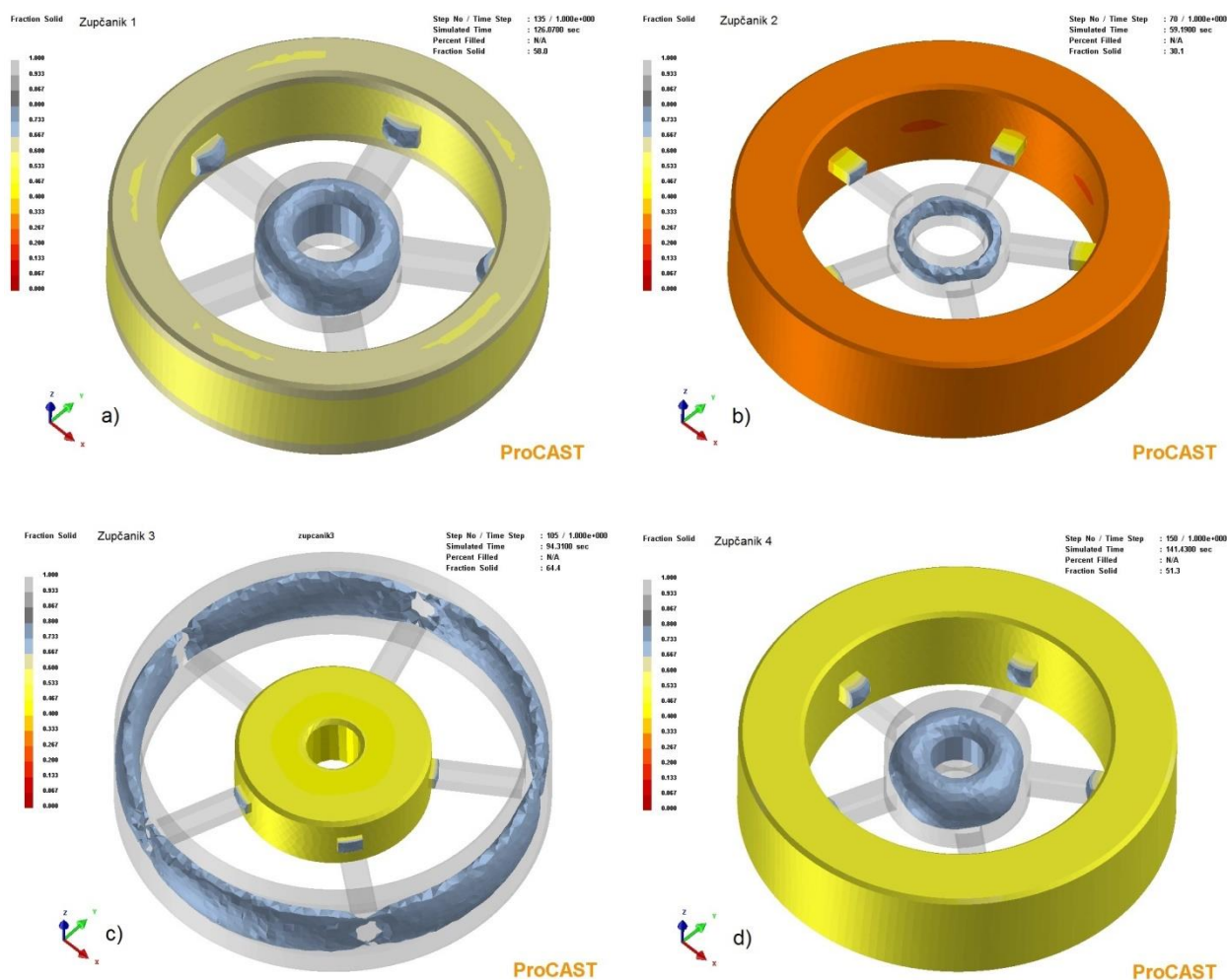
Slika 51. Kraj skrućivanja špica zupčanika te početak vijenca i glavine
