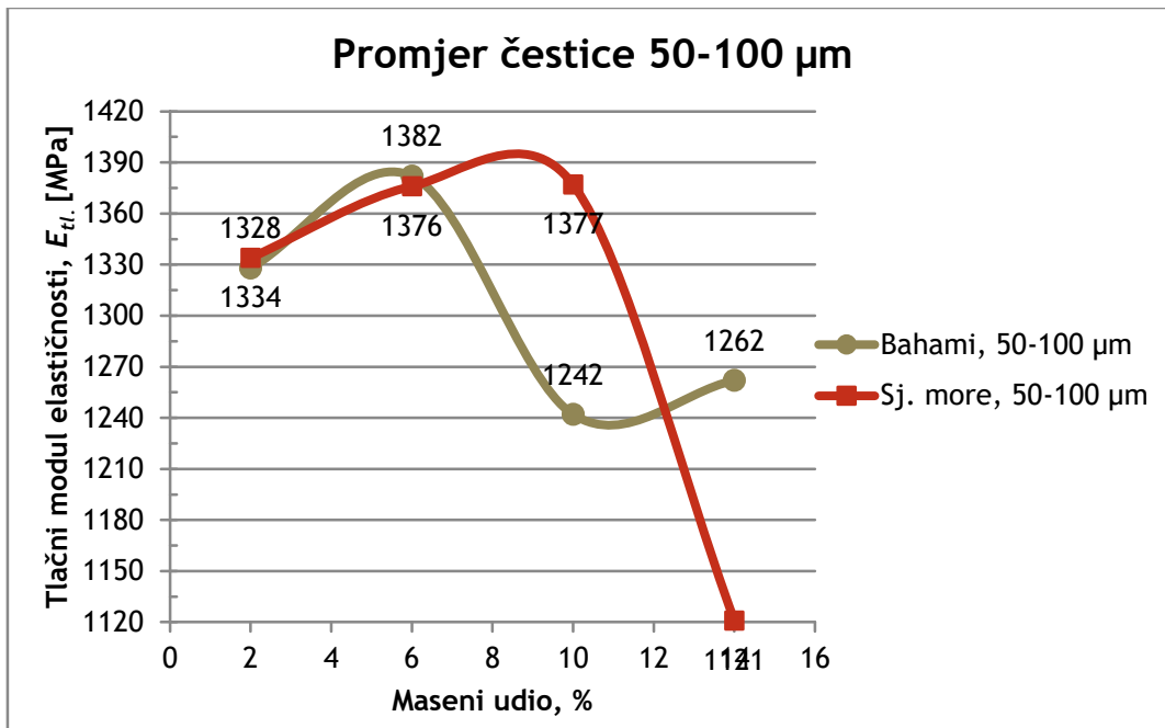
Slika 40. Modul elastičnosti uzoraka s promjerom čestice 50-100 μm
