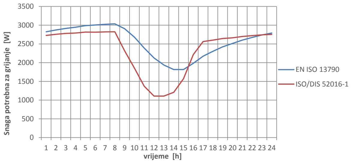
Dijagram 34. Rezultati potrebne snage za grijanje za uprosječni dan u prosincu prema ISO/DIS 52016-1 i EN ISO 13790
