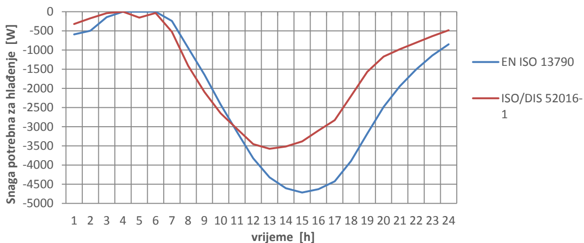
Dijagram 43. Rezultati potrebne snage za hlađenje za uprosječni dan u srpnju prema ISO/DIS 52016-1 i EN ISO 13790 prema 4. slučaju
