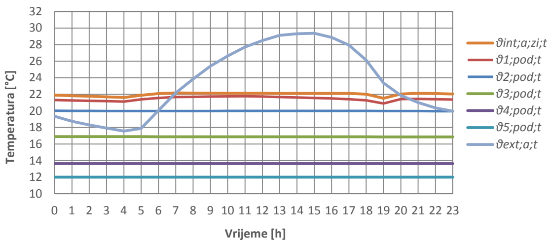
Dijagram 28. Dnevne raspodjele temperatura svih čvorova poda za uprosječni dan u kolovozu
