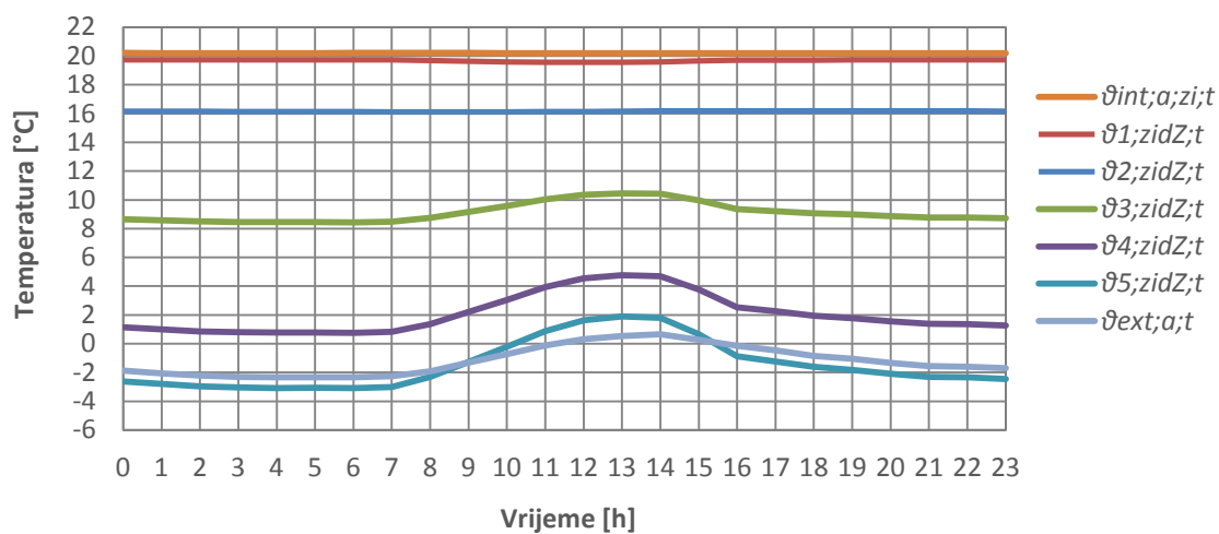
Dijagram 6. Dnevne raspodjele temperatura svih čvorova vanjskog zida orijentiranog prema zapadu za uprosječni dan u siječnju
