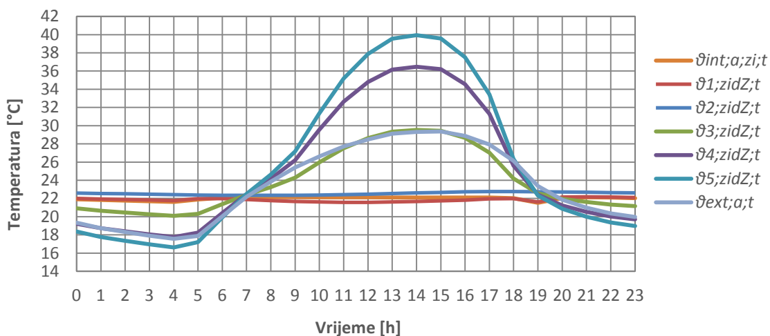
Dijagram 25. Dnevne raspodjele temperatura svih čvorova vanjskog zida orijentiranog prema zapadu za uprosječni dan u kolovozu
