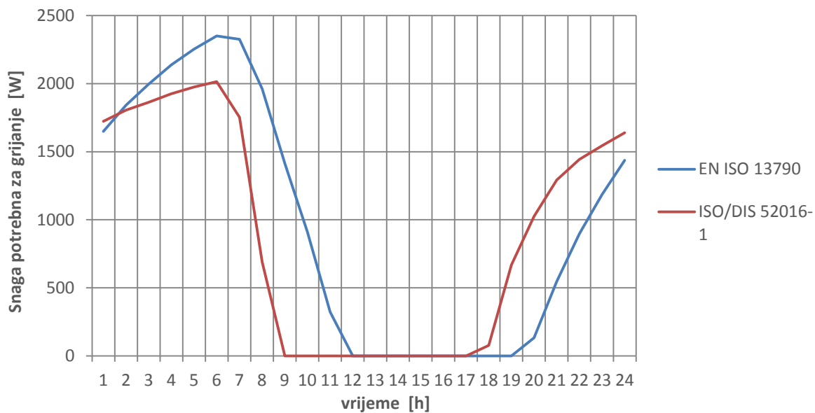
Dijagram 15. Rezultati potrebne snage za grijanje za uprosječni dan u ožujku prema ISO/DIS 52016-1 i EN ISO 13790
