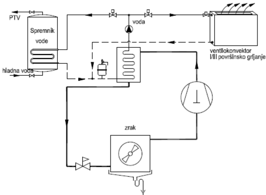
Slika 2.7. Dizalica topline zrak-voda [3]
