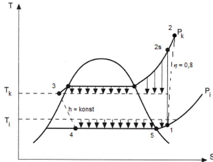
Slika 5.2. Termodinamički proces dizalice topline u T-s dijagramu
