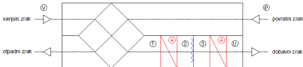
Slika 13. Osnovne komponente klimatizacijske jedinice
