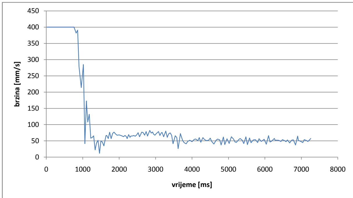
Slika 47: Brzina robota
