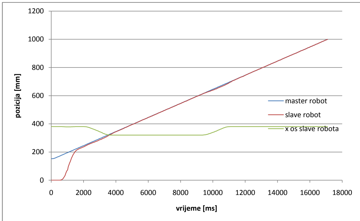
Slika 49: Putanja slave i master robot
