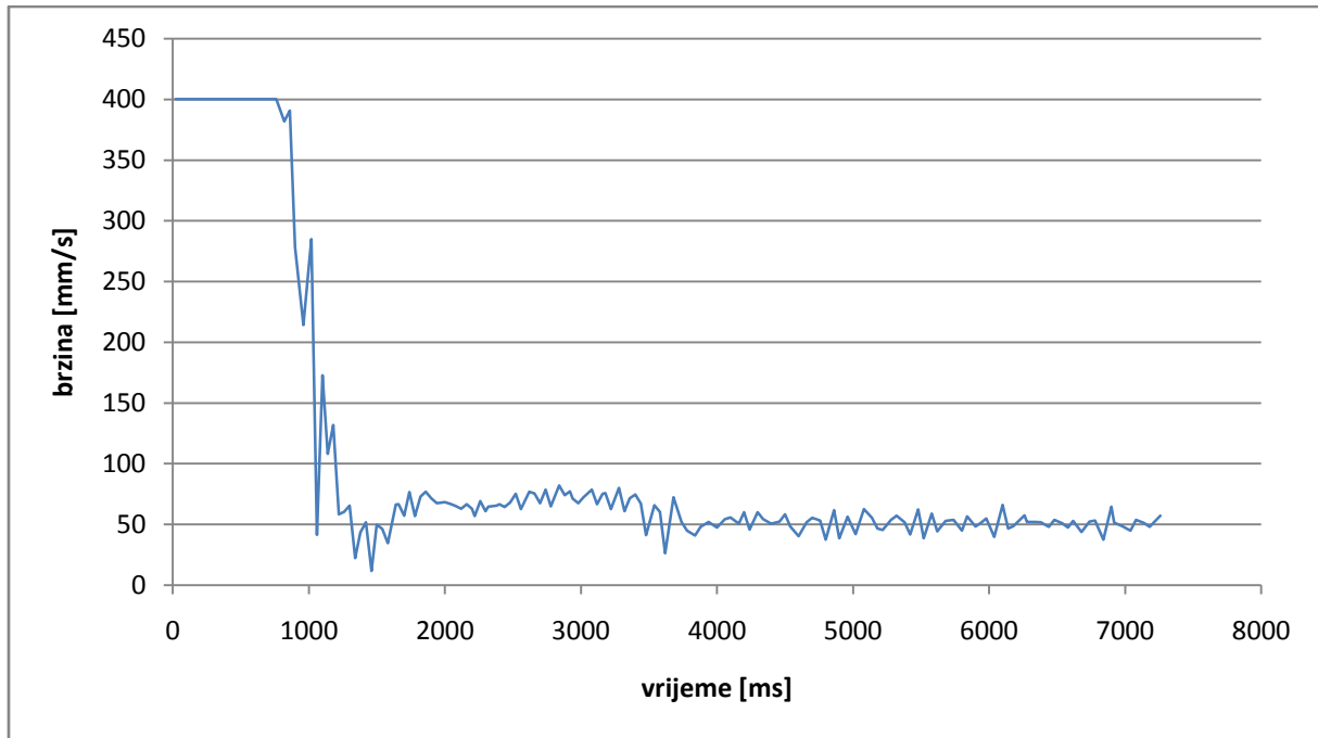
Slika 47: Brzina robota
