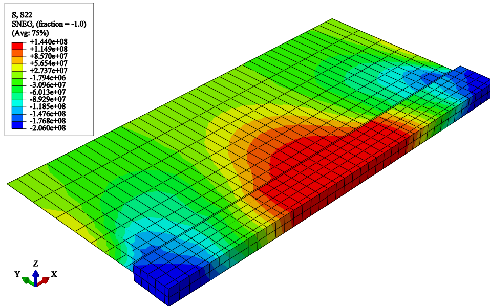
Slika 88. Raspodjela transverznog napreznja \sigma_y (N/m 2 ) na 3D/ljuskastom modelu širine 3D zone 2,5t analiziranog pomoću AWI – a
