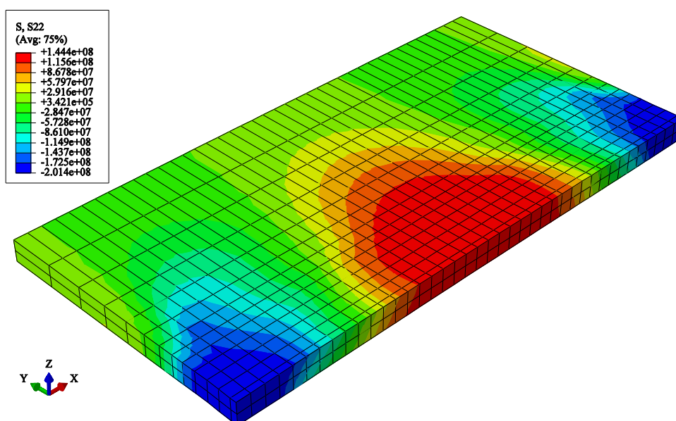
Slika 42. Raspodjela transverznog napreznja \sigma_y ( \text{N/m}^2 ) na 3D modelu
