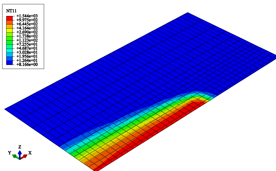
Slika 32. Temperaturno polje na ljuskastom modelu početkom 11. sekunde drugog prolaza elektrode, T ( ^{\circ}\text{C} )
