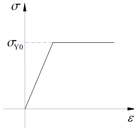
Slika 4. Elastičan-idealoplastičan materijalni model [6]
