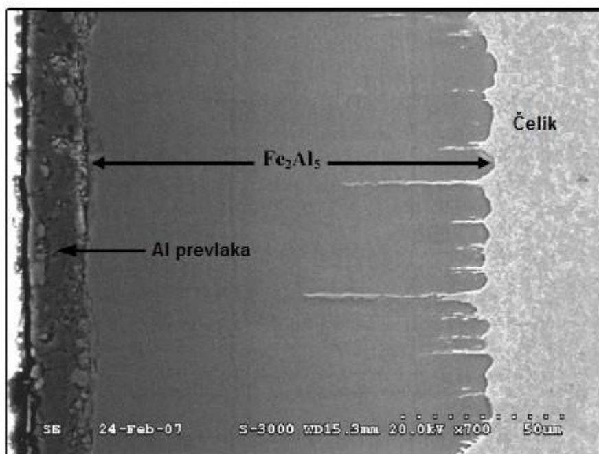
Slika 21. Mikrostruktura srednje ugljičnog čelika nakon aluminiziranja uranjenjem u čistu taljevinu aluminija na 30 minuta i poliranjem površine obratka u 2% Nitalu
