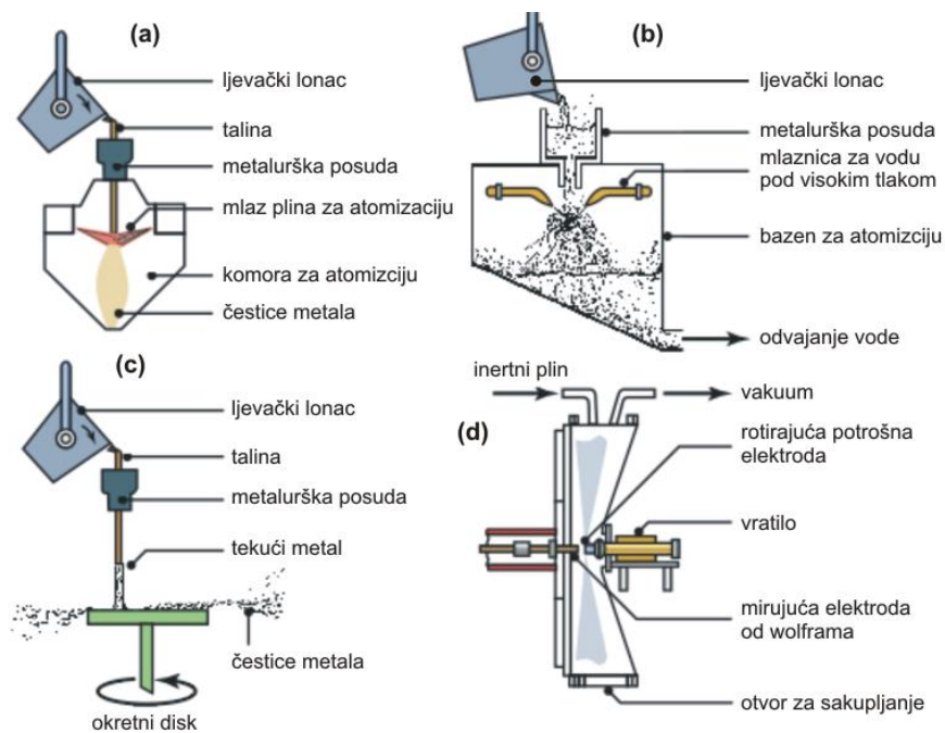
Slika 5. Postupci atomizacije [9]
