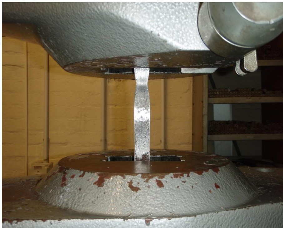
Slika 59. Ispitni uzorak u čeljustima kidalice [29]
