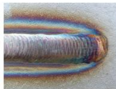
b) Obojenja površine nastala unosom topline zavarivanjem
