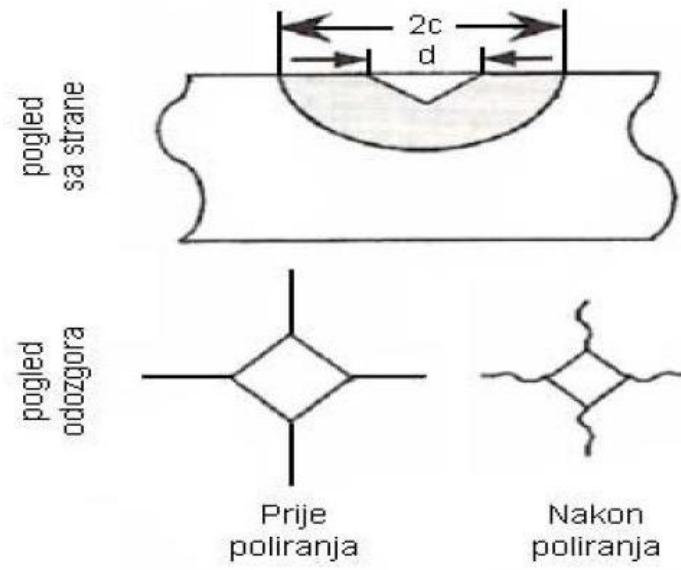
Slika 17. Medijan pukotina [15]
